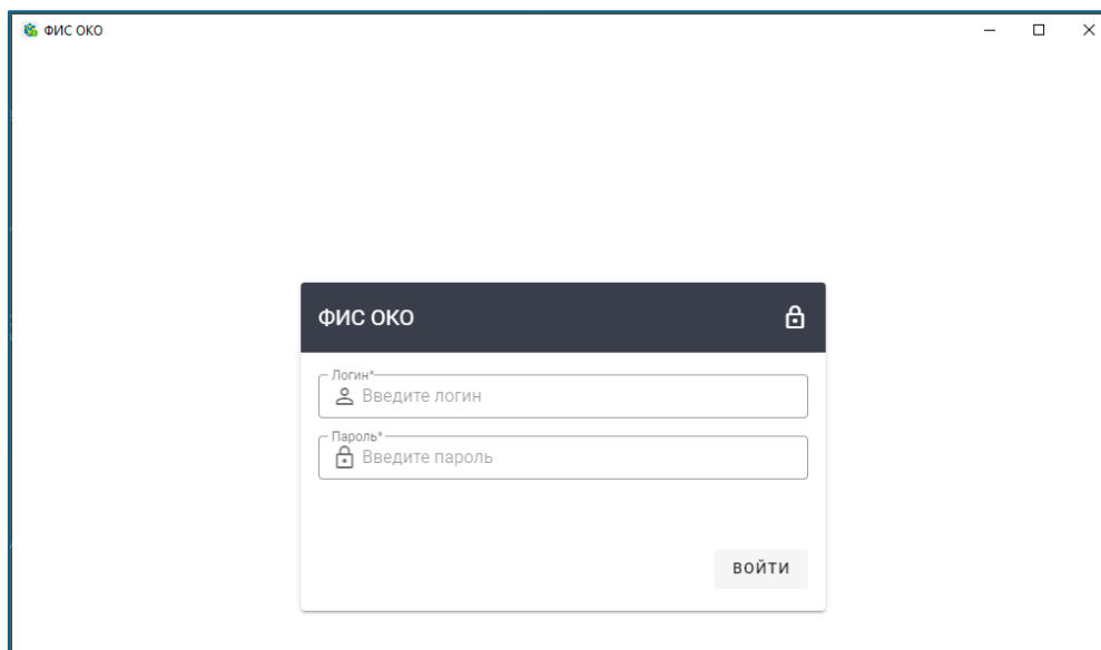
Рис.2. Окно авторизации
